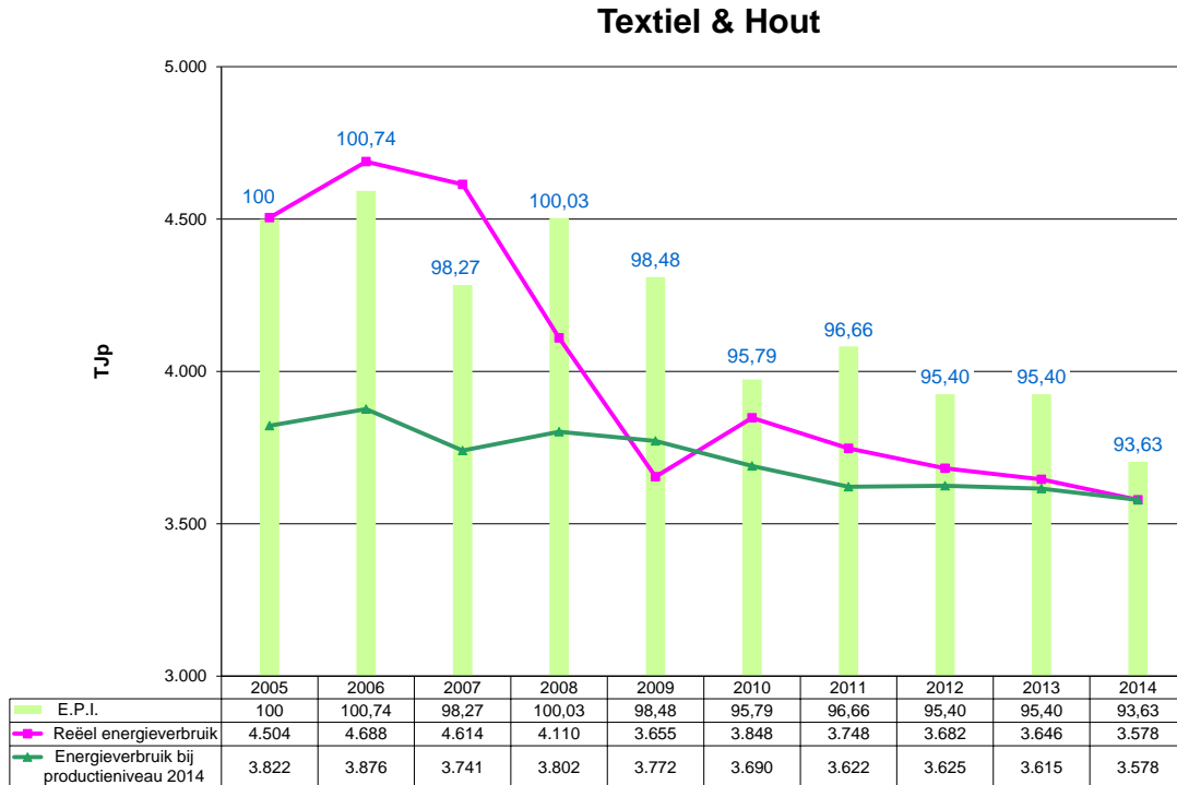
Grafiek 5 : Evolutie 2005 - 2014 van het primaire energieverbruik en de E.P.I. voor de Textiel- en Houtbedrijven
