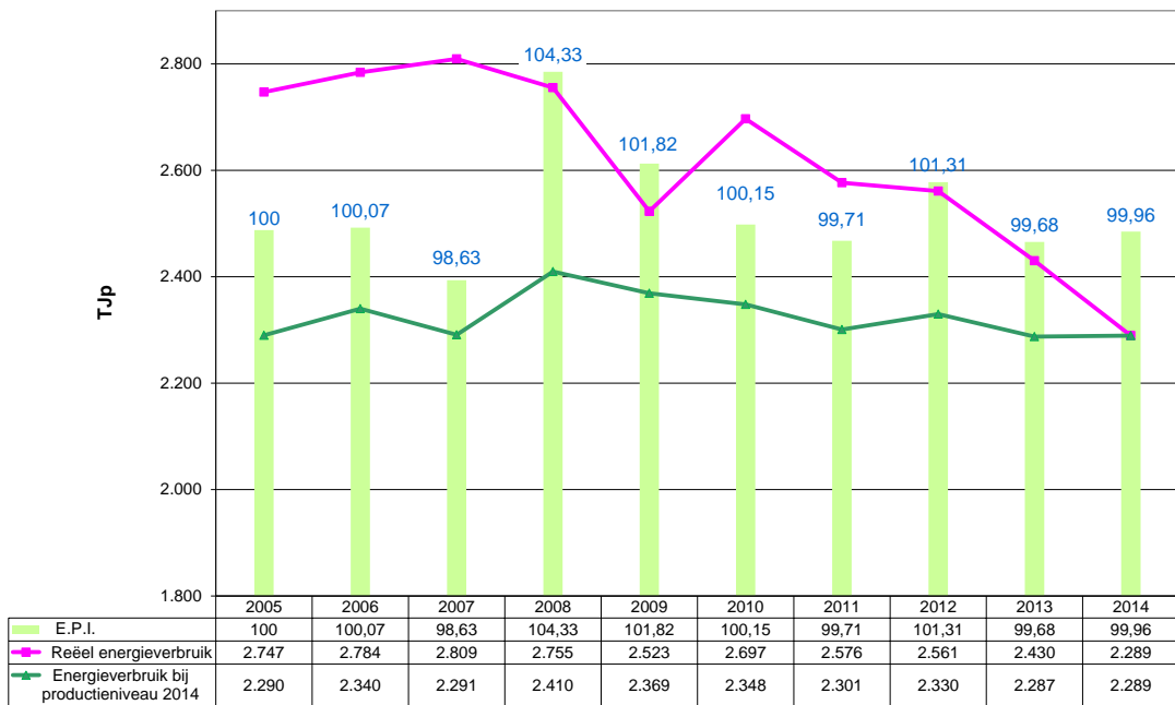
Grafiek 6 : Evolutie 2005 - 2014 van het primaire energieverbruik en de E.P.I. voor de bedrijven uit de groep Diversen (Minerale producten, Glas, Papier- en kartonverwerking en de Grafische sector)
