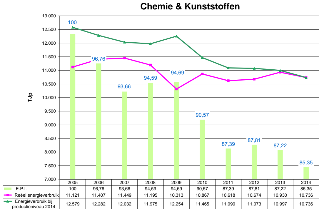
Grafiek 2 : Evolutie 2005 - 2014 van het primaire energieverbruik en de E.P.I. voor de Chemie- en Kunststoffverwerkende bedrijven
