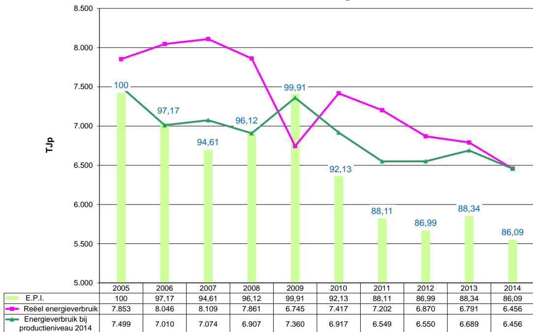
Grafiek 4 : Evolutie 2005 - 2014 van het primaire energieverbruik en de E.P.I. voor de Technologiebedrijven
