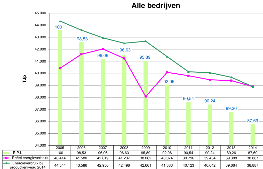
Grafiek 1 : Evolutie 2005 - 2014 van het energieverbruik en de E.P.I. voor alle bedrijven
