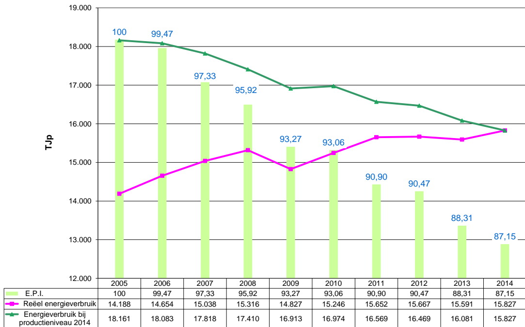
Grafiek 3 : Evolutie 2005 - 2014 van het primaire energieverbruik en de E.P.I. voor de Voedings- en Mengvoederbedrijven
